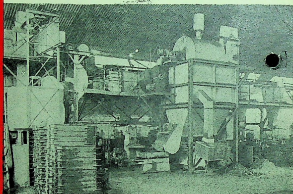
Sistema mecanizado de preparación, transporte y moldeo neumático de las arenas de fundición, lo que asegura un producto homogéneo y una economía de fabricación.
