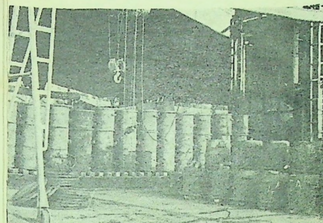
Parte de la sección de tratamientos térmicos para la fundición de hierro maleable en que puede verse el Horno y el carro cargado con cajas selladas que contienen las piezas por maleabilizar.
