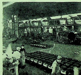
Sistema mecanizado de preparación, transporte y moldeo neumático de las arenas de fundición, lo que asegura un producto homogéneo y una economía de fabricación.
